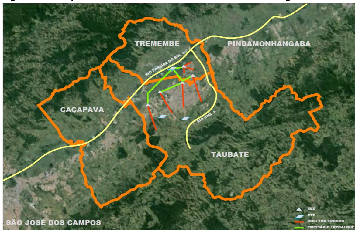
Figura 3 – Compartilhamento do Sistema de Tratamento de Esgotos
