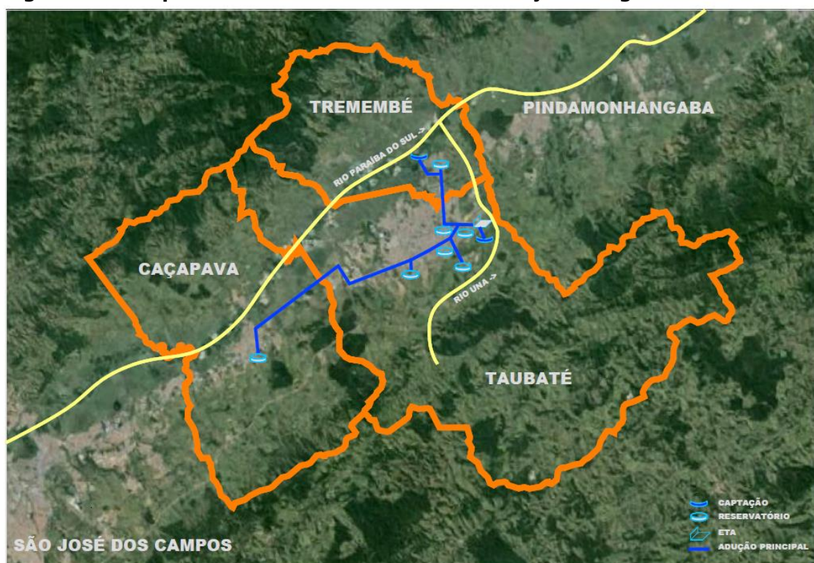
Figura 2 – Compartilhamento do Sistema de Produção de Água
